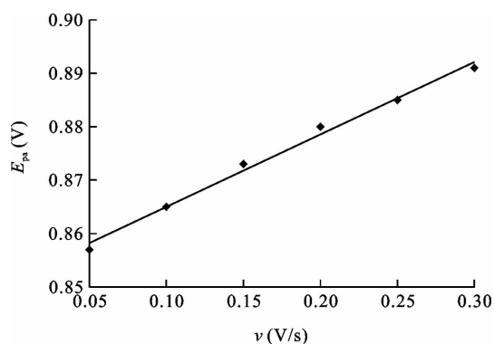
图 7 E_{pa} 与扫速 v 的关系
