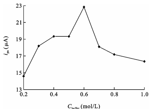
图 9 MG 的 i_{pa} 与 PBS 浓度关系
