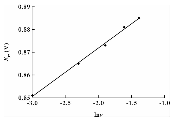
图 6 E_{pa} 与 \ln v 的关系
