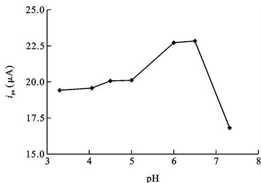
图 8 MG 的 i_{pa} 与 pH 值关系
