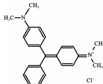
图1 MG 的结构式
